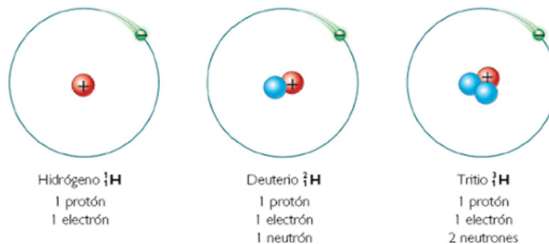
Fig.10. Isótopos naturales del hidrógeno.
