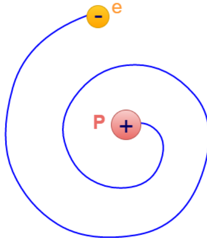
Fig. 18. El modelo planetario no era coherente con la física conocida hasta el momento, ya que según este, el electrón colapsaría al núcleo.
