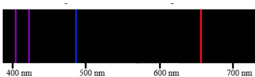
Figura 20. Espectro de emisión del hidrógeno al ser calentado
