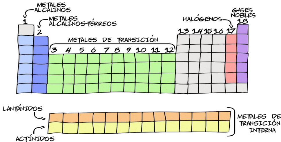
Fig X. Algunas familias y subtipos de elementos
