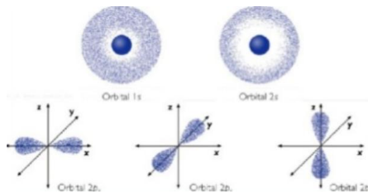
Fig.12: Modelo atómico actual extraído de http://ventosdouniverso.blogspot.com/2012/02/sumario-para-o-blogonauta-1.html
