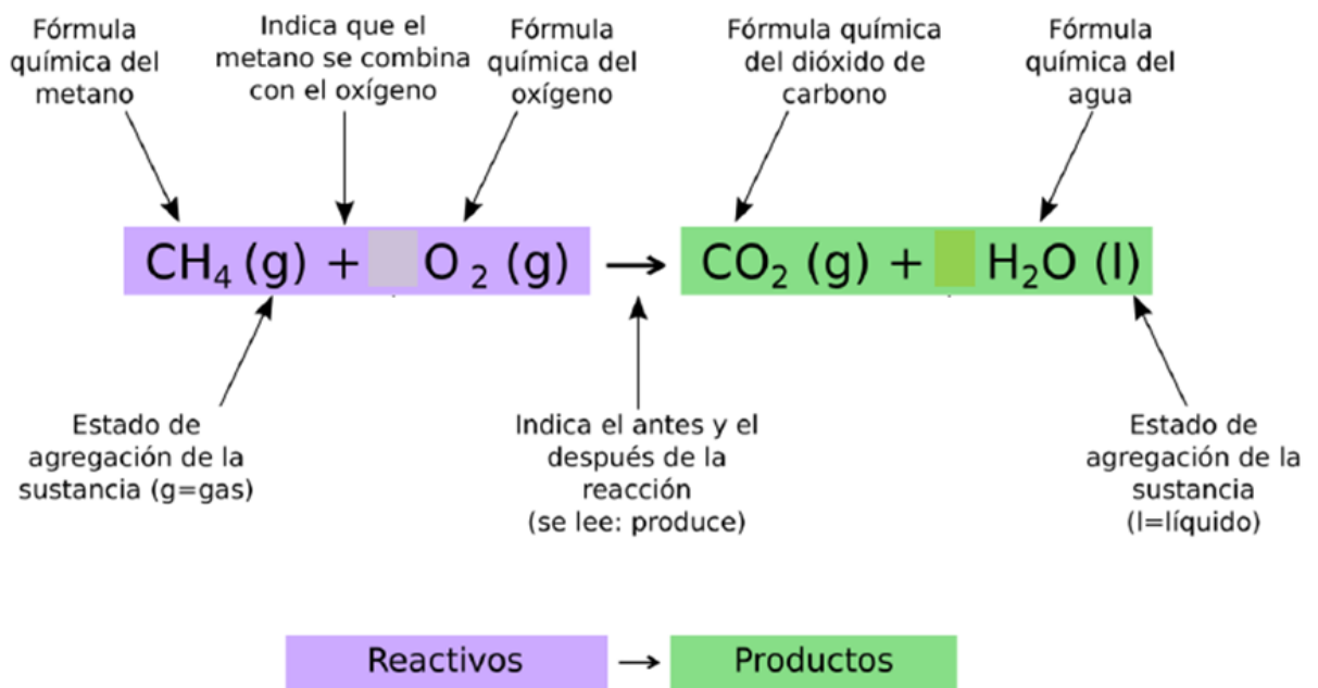
Fig.7: Ejemplo de una reacción de combustión completa del gas metano
