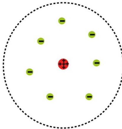
Fig. 17. El modelo nuclear de Rutherford
