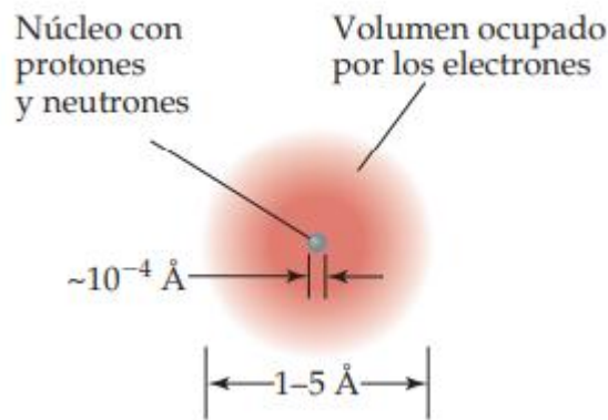
Fig.9: Tamaños relativos del átomo y su núcleo. Extraído de Brown (2004).
