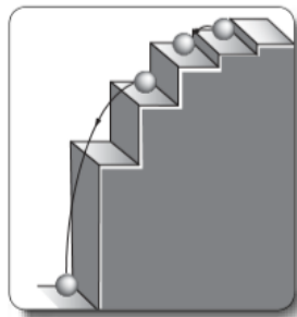
Figura 19. Como la posición de una pelota en una escalera: la pelota no puede situarse entre los escalones, lo mismo ocurre con los electrones.
