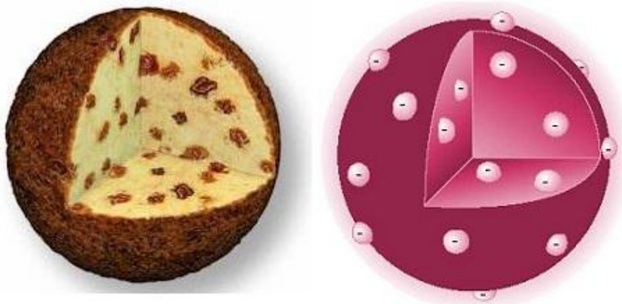
Fig. 13. Modelo del budín de pasas y modelo de Thomson
