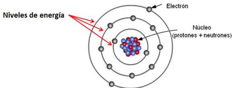
Fig.11. Modelo atómico de Bohr
